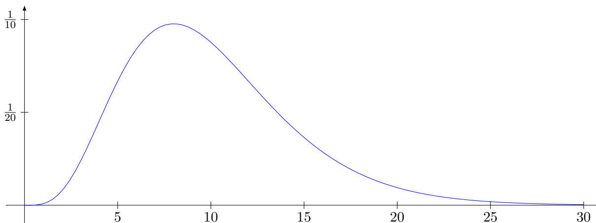
FIGURE 36.1: La densité de \chi^2(10) .
