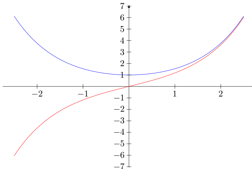
FIGURE 42.1: En rouge, la fonction x \mapsto \sinh(x) et en bleu, la fonction x \mapsto \cosh(x) . LabelFigsYNRaoZBuEWsWw
