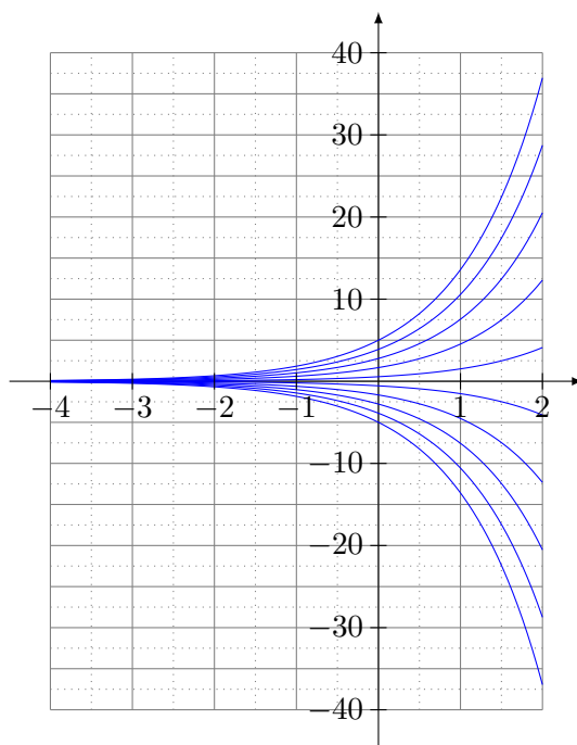
FIGURE 32.1: Quelques trajectoires de l'équation y' = y .
