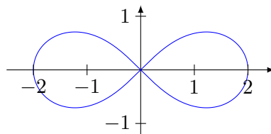
FIGURE 20.10: Intégrer sur des domaines plus complexes. LabelFigPONXooXYjEot
