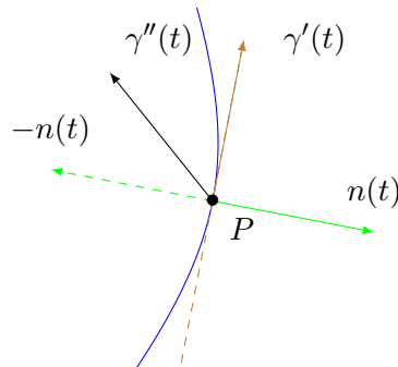
FIGURE 21.9: De quel côté de \gamma'(t) se trouvent n(t) et -n(t) ?
