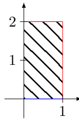
FIGURE 20.6: Intégration sur un rectangle
