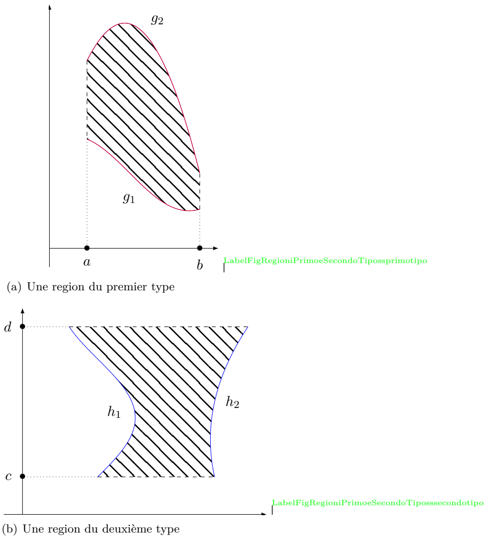
FIGURE 20.17: Régions du premier et du deuxième type
