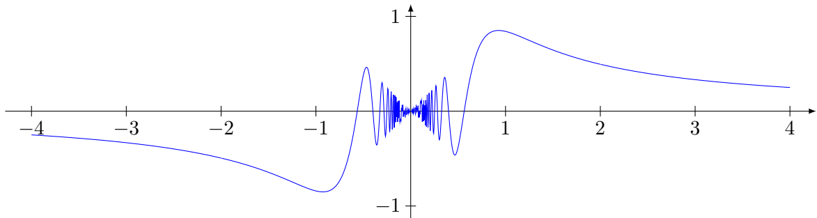
FIGURE 18.11: La fonction de l'exemple 18.246.
