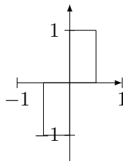
FIGURE 18.8: Le compact K et son image par R_0(\pi) pour le lemme 18.211.
