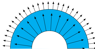
FIGURE 12.16: Le champ de vecteur de la gravité. Nous avons tracé, sur les deux cercles la même densité de vecteurs, c'est-à-dire le même nombre de vecteurs par unité de surface. LabelFigZGUDooEsqCWQ
