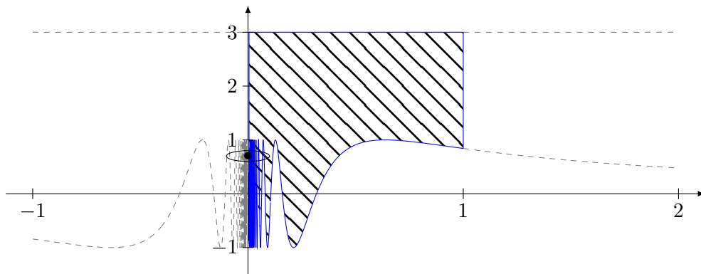
FIGURE 9.2: Les points qui sont sur l'axe vertical entre 0 et 3 sont sur la frontière, mais pas dans l'ensemble A_5 .
