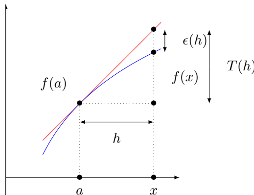
FIGURE 12.10: Interprétation géométrique de la différentielle. LabelFigDifférentielle
