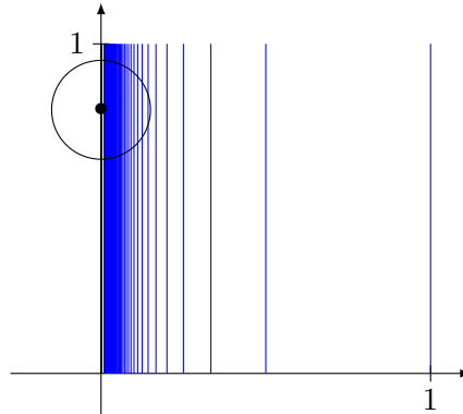
FIGURE 9.3: Le segment sur l'axe vertical entre y = 0 et y = 1 fait partie de l'adhérence et de la frontière, mais pas de l'ensemble A_6 lui-même.
