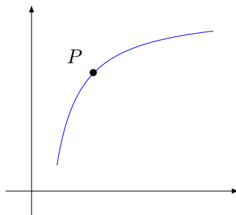
FIGURE 12.1: Comment trouver la tangente à la courbe au point P ? LabelFigTangenteQuestion
