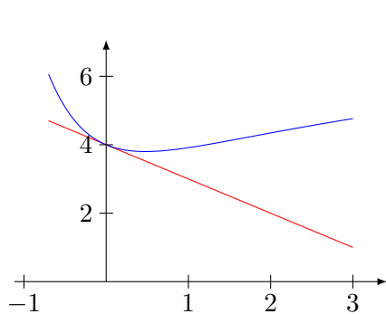
(a) Polyôme d'ordre 1
