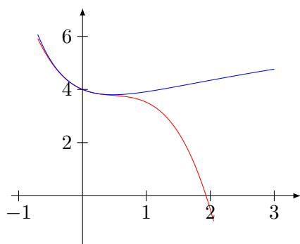
(c) Polyôme d'ordre 3
