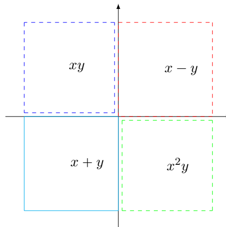
FIGURE 12.11: La fonction de l'exemple 12.264.
