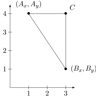
FIGURE 10.1: La norme euclidienne induit la distance euclidienne. D'où son nom. Le point C est construit aux coordonnées (A_x, B_y) .
