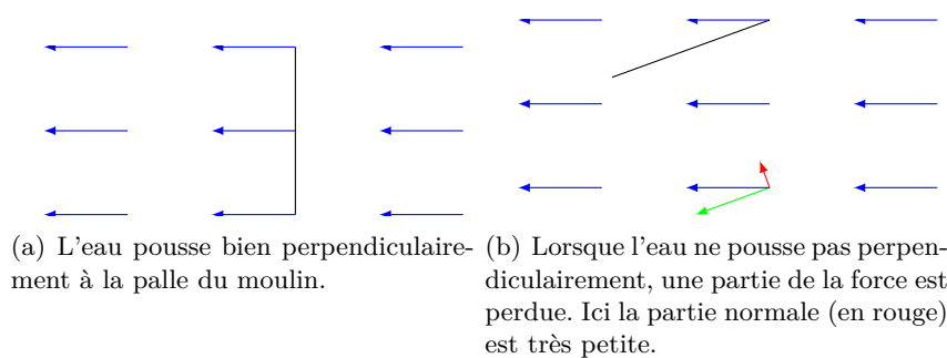
FIGURE 20.2 – La partie rouge de la force est perdue si l'eau ne pousse pas perpendiculairement. De plus lorsque la pale est inclinée, elle prend moins d'eau sur elle.
