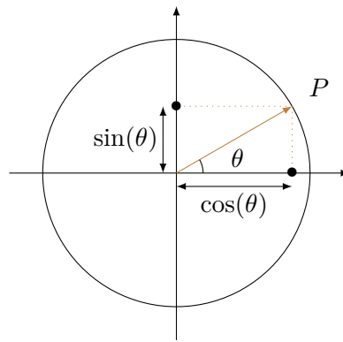
FIGURE 18.6 – Le cercle trigonométrique.
