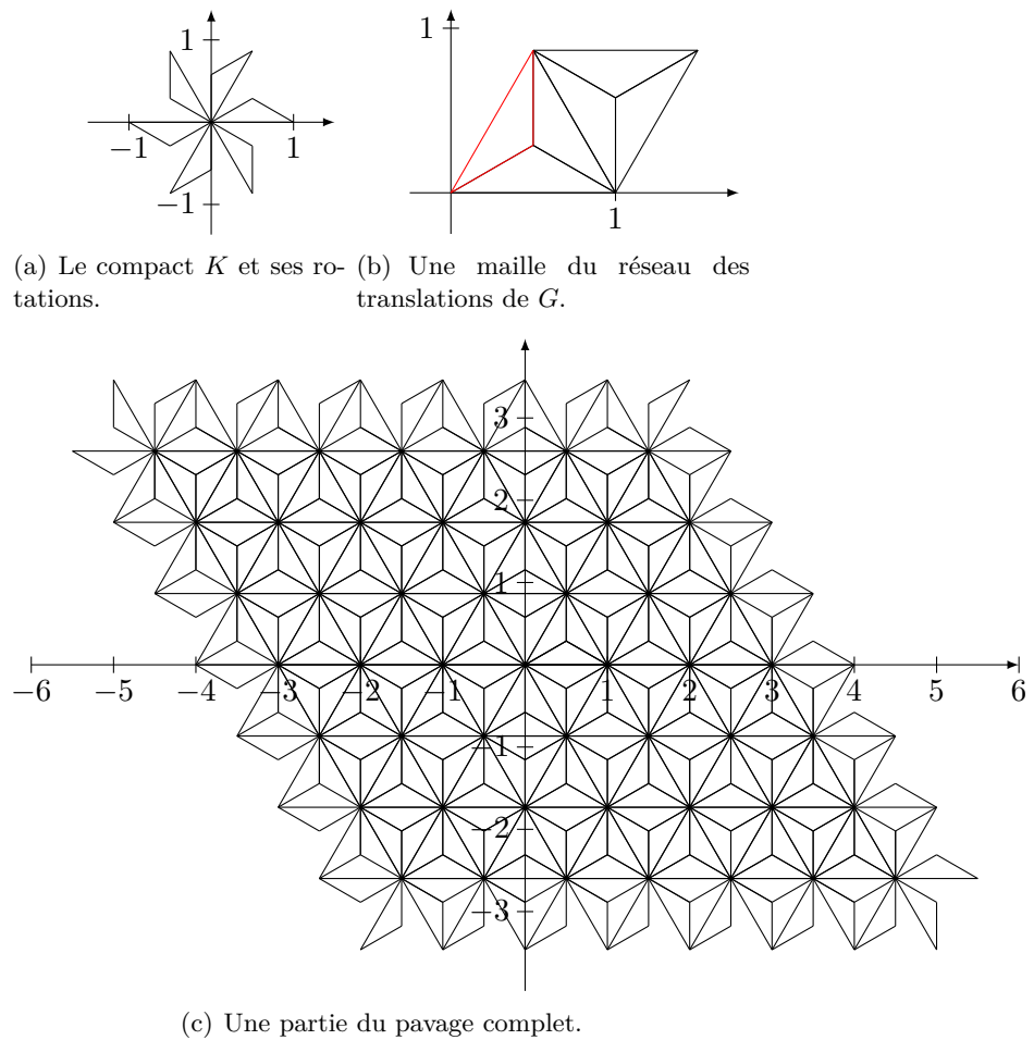
FIGURE 18.10 – Illustrations pour le pavage du lemme 18.188.
