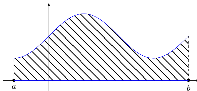
FIGURE 20.5 – L'intégrale de f entre a et b représente la surface sous la fonction.
