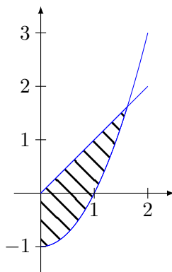
FIGURE 20.18 – La région A de l'exemple 20.187
