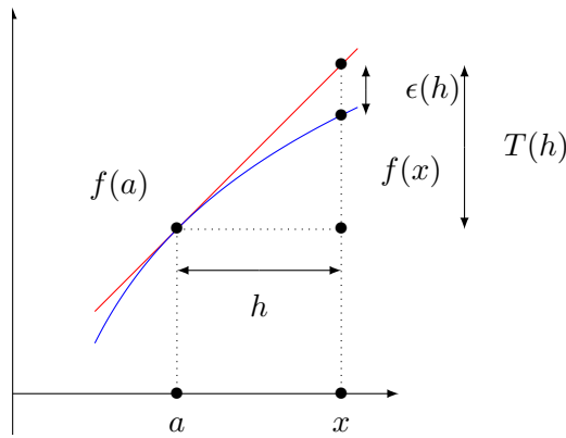
FIGURE 12.10 – Interprétation géométrique de la différentielle.
