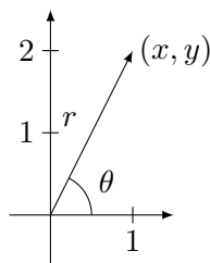
FIGURE 18.11 – Un point en coordonnées polaires est donné par sa distance à l'origine et par l'angle qu'il faut avec l'horizontale.
