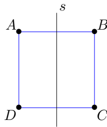
FIGURE 18.8 – Le carré dont nous étudions le groupe diédral.
