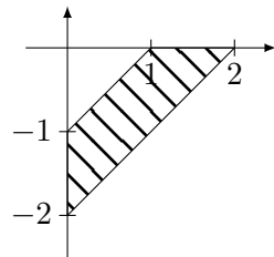
(a) La région V
