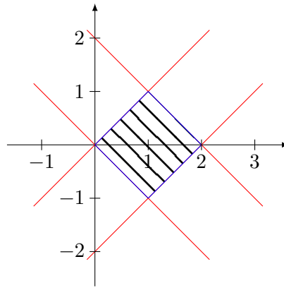
FIGURE 18.15 – Un domaine qui s’écrit étonnamment bien avec un bon changement de coordonnées.
