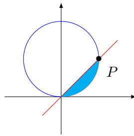
FIGURE 18.14 – Passage en polaire pour intégrer sur un morceau de cercle.
