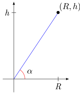
FIGURE 18.16 – En faisant tourner cette droite autour de l'axe X , nous obtenons un cône.
