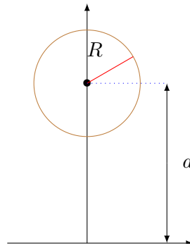
FIGURE 18.17 – Si nous tournons ce cercle autour de l’axe X , nous obtenons un tore de rayon « externe » a et de rayon « interne » R .
