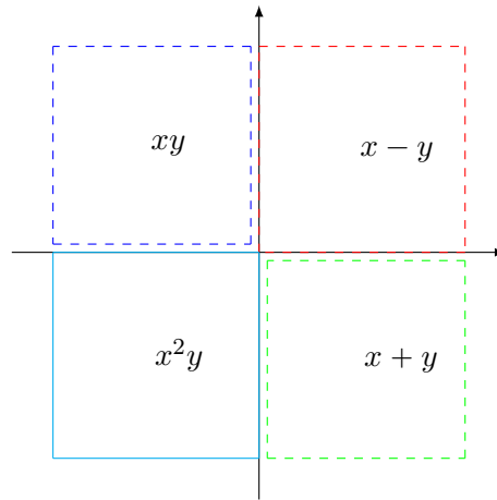
FIGURE 12.11 – La fonction de l'exemple 12.223.
