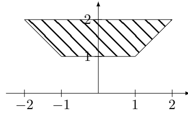
(b) La région U = \phi^{-1}(V)
