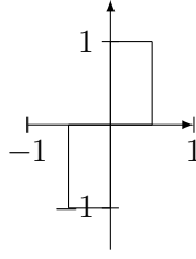
FIGURE 18.9 – Le compact K et son image par R_0(\pi) pour le lemme 18.186.
