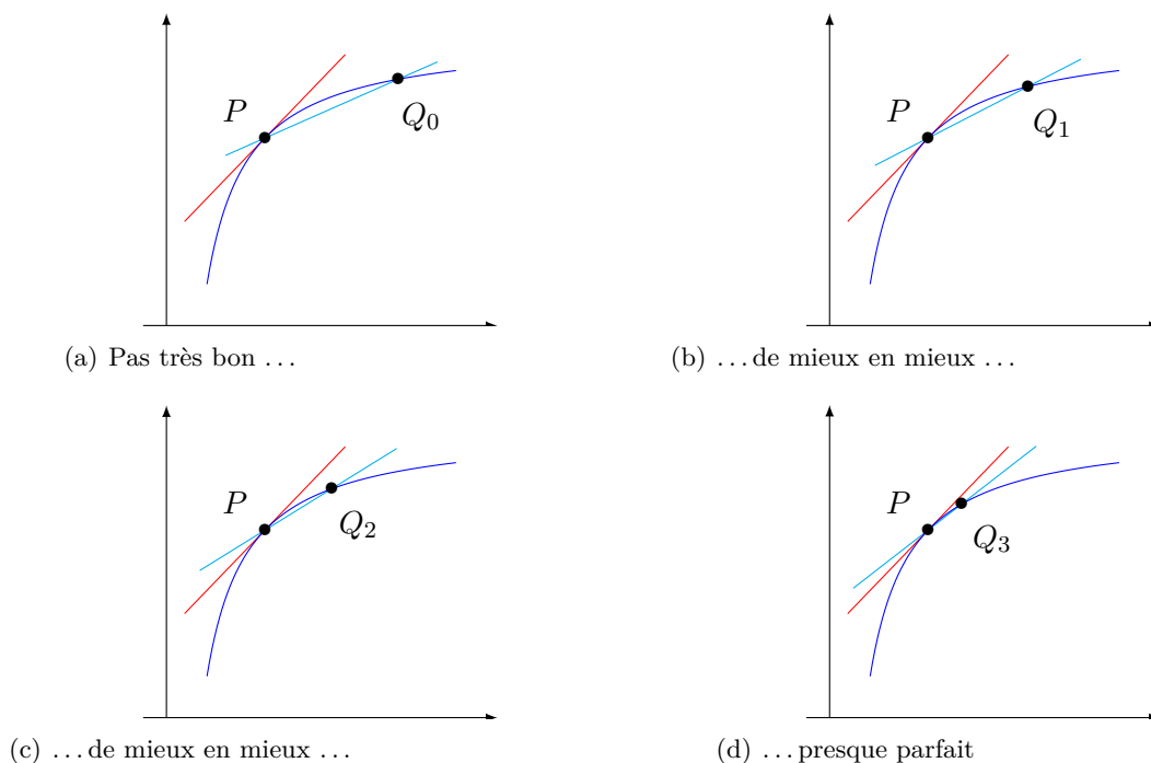
FIGURE 12.3 – Recherche de la tangente par approximations successives.
