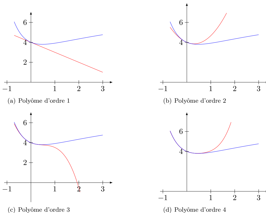
FIGURE 12.12 – Les développements limités d'ordre de plus en plus grand de la fonction de l'exemple 12.417. La fonction est en bleu et les « approximations » sont en rouge.
