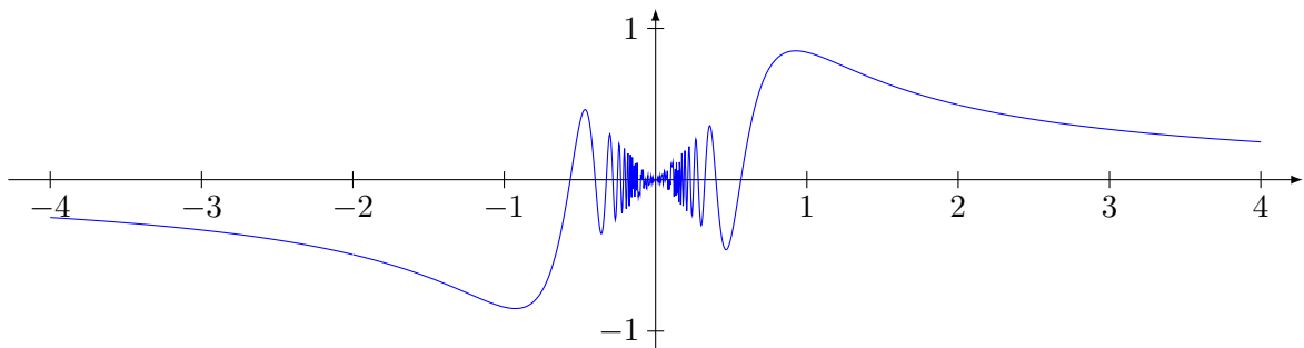
FIGURE 18.12 – La fonction de l'exemple 18.220.
